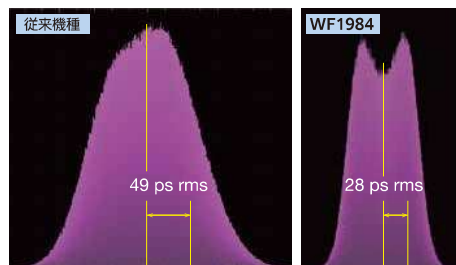
方形波, 1.11 MHz, 2 V p-p / 50 Ω
