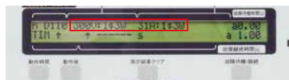
電圧レンジおよび電流レンジの設定
