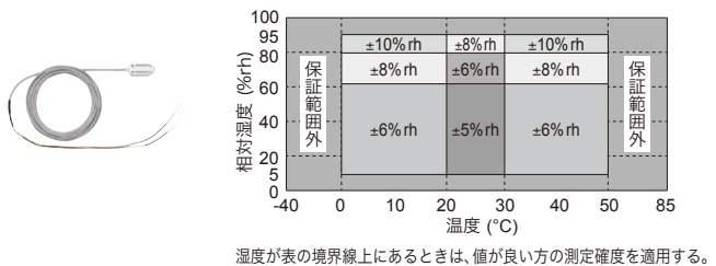
湿度センサ Z2000 使用時精度表
