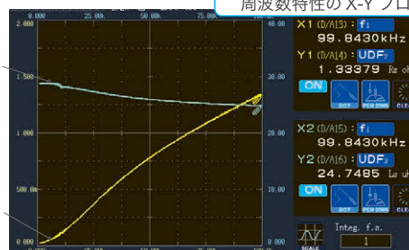
リアクトルのインピーダンス - 周波数特性の X-Y プロット
