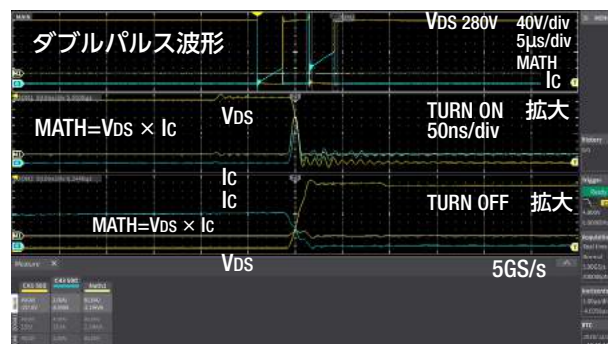
パワーデバイス (GaN) のダブルパルス波形ターンONとターンOFF波形を拡大表示
