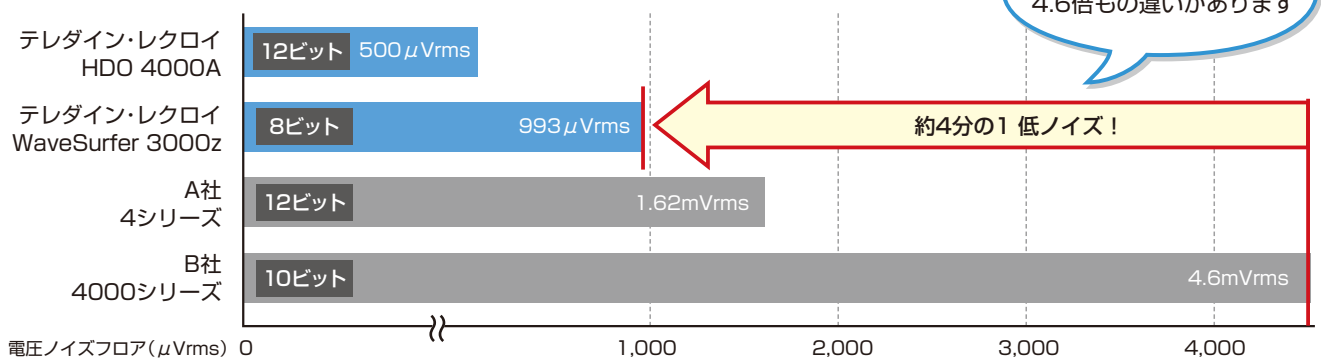
1GHz製品の電圧ノイズフロア比較
